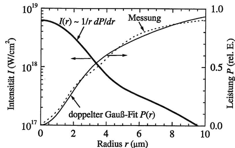
Abbildung 3.3: Eingeschlossene Leistung (Messung als gestrichelte und Fit als dünne durchgezogene Linie) und Intensität im Fokus (dicke durchgezogene Linie). Die waagrechten Pfeile deuten auf die Ordinate der jeweiligen Kurve.
