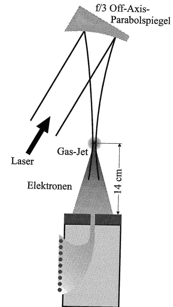
Abbildung 4.9: Einsatz des Elektronenspektrometers im Experiment.
