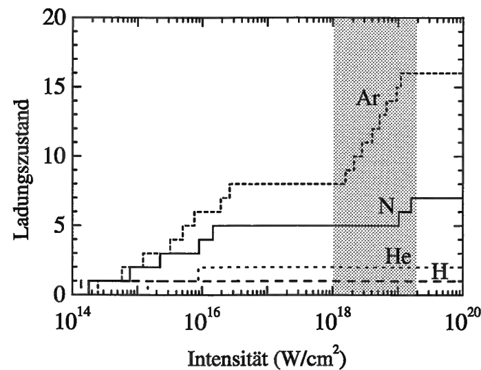
Abbildung 5.9: Ionisationszustand für verschiedene Elemente in Abhängigkeit von der eingestrahlt Laserintensität. Der im Kanal erreichte Intensitätsbereich ist grau unterlegt.
