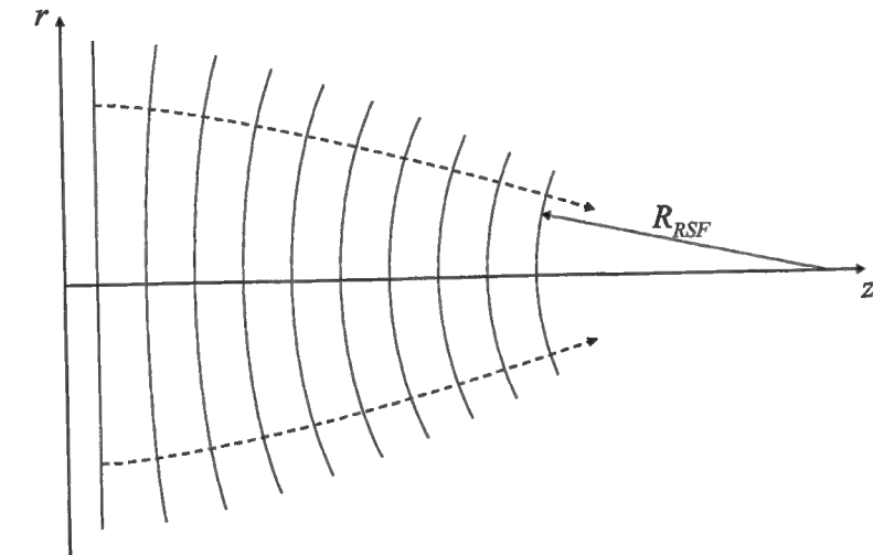
Abbildung 2.5: Einfluß des nichtlinearen Brechungsindex \eta_2 > 0 auf die Wellenfronten (durchgezogene Linien) und deren Normalen (gestrichelte Linien). Der Krümmungsradius R_{RSF} einer Wellenfront ist als gepunkteter Pfeil dargestellt.
