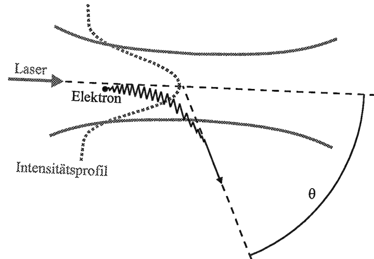
Abbildung 2.1: Prinzip der ponderomotorischen Streuung eines Elektrons im Laserfokus.
