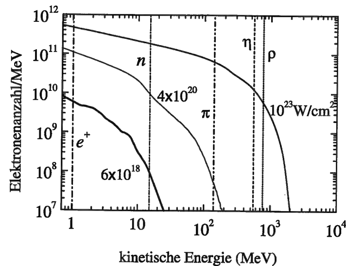
Abbildung 8.1: Elektronenspektren (durchgezogene Linien) für unterschiedliche Laserintensitäten (in normalen Lettern). Das Spektrum für 6 \times 10^{18} \text{ W/cm}^2 ist das gemessene aus Abb. 5.7, die anderen beiden Spektren resultieren aus PIC-Simulationen [90]. Die senkrechten Linien entsprechen den Schwellenenergien zur Erzeugung der angezeigten Elementarteilchen.
