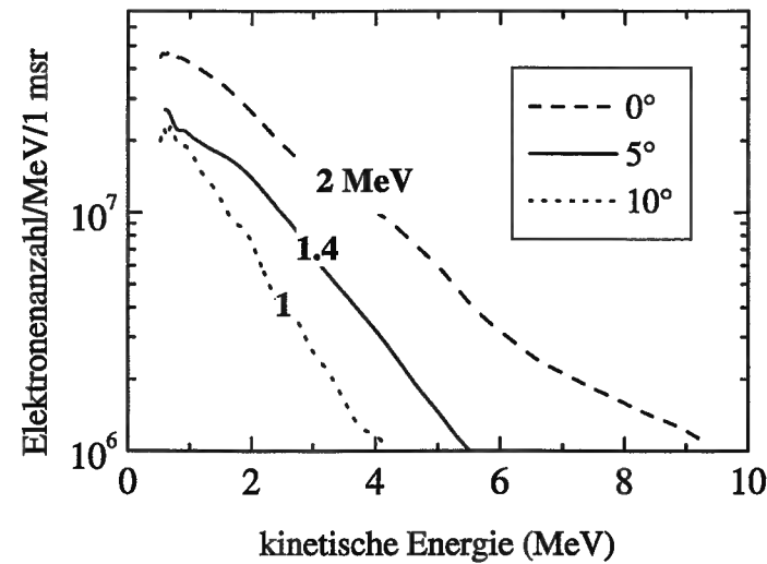
Abbildung 5.5: Spektrale Verteilung der Elektronen in Abhängigkeit vom Winkel relativ zur Laserachse ( n_e = 10^{20} \text{ cm}^{-3} ). Angabe der effektiven Temperatur der (nicht gezeigten) angepaßten Exponentialkurven in fetten Lettern.
