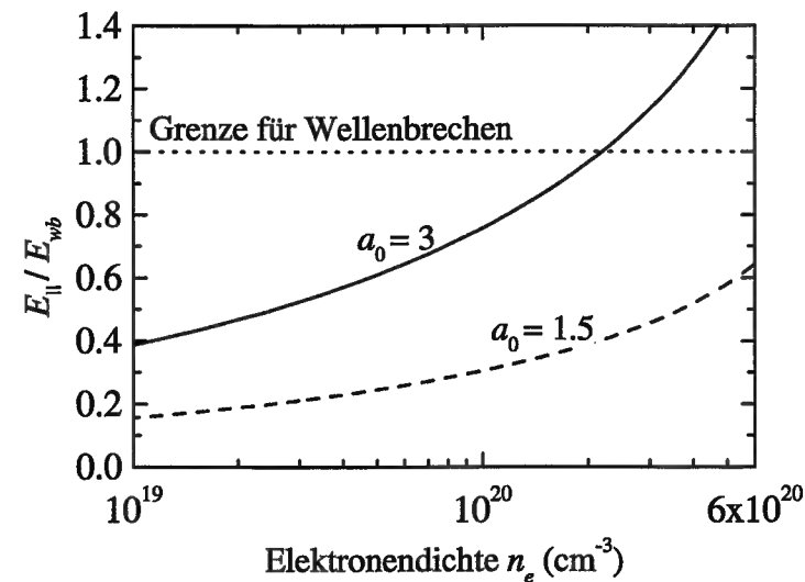
Abbildung 2.9: Feldamplitude der Welle E_{||}/E_{wb} in Abhängigkeit von der Plasmadichte bei LWFA für a_0 = 1.5 (gestrichelte Linie) und a_0 = 3 (durchgezogene Linie). Die gepunktete Linie stellt die Grenze dar, oberhalb derer Wellenbrechen einsetzt.
