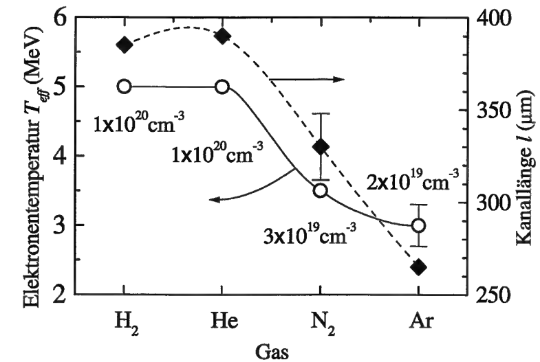
Abbildung 5.10: Kanallänge (gefüllte Rauten) und Temperatur (offene Kreise) für verschiedene Gassorten. Die Fehlerbalken resultieren aus Schuß-zu-Schuß-Schwankungen, die Linien dienen nur als visuelle Hilfe. Die Pfeile deuten auf die Ordinate der jeweiligen Kurve. Zusätzlich sind die atomaren bzw. molekularen Dichten im Jet angezeigt.
