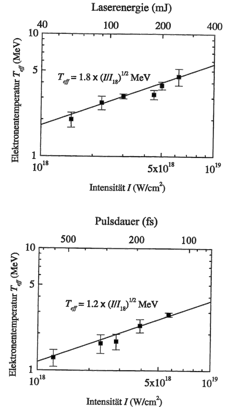
Abbildung 5.8: Effektive Elektronentemperatur in Abhängigkeit von der (im Vakuum gemessenen) Laserintensität ( n_e = 2 \times 10^{20} \text{ cm}^{-3} ) bei Variation der Laserenergie (oben) bzw. der Pulsdauer (unten). Die am besten angepaßte Kurve ergibt die jeweils angegebene Skalierung mit I_{18} = 10^{18} \text{ W/cm}^2 .
