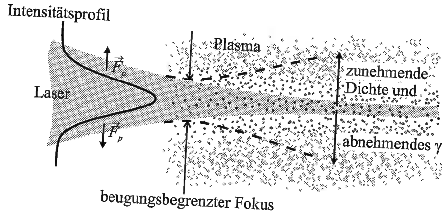
Abbildung 2.2: Prinzip der Selbstfokussierung in einem unterdichten Plasma. Die Punkte stellen Elektronen dar. Je dunkler sie sind, desto höher ist ihr relativistischer \gamma -Faktor. Die gestrichelten Linien deuten die Strahlteile im Vakuum an, \vec{F}_p ist die ponderomotorische Kraft.
