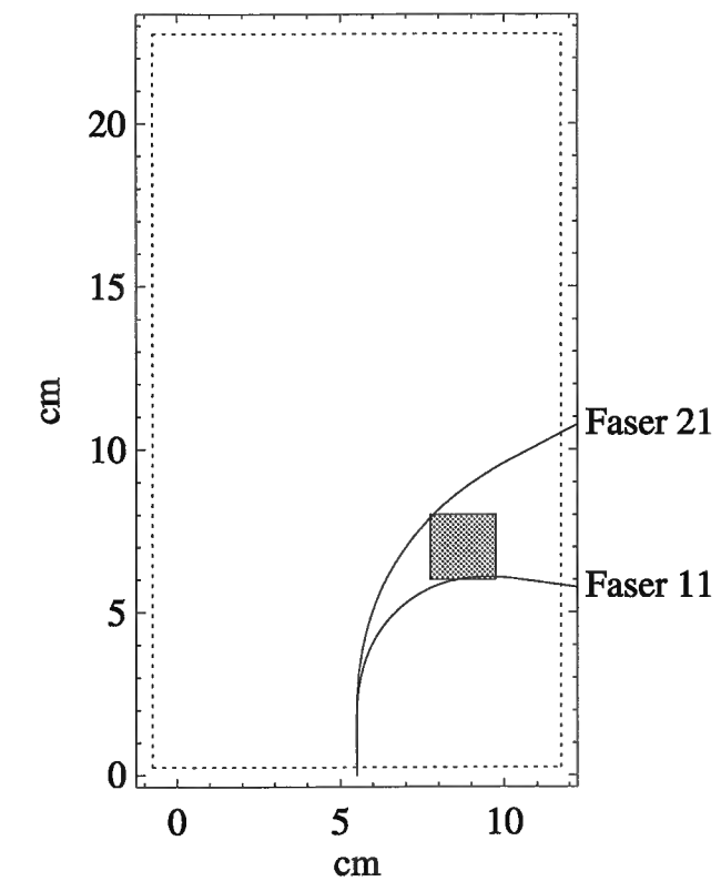
Abbildung 4.11: Position des Plastikblocks (kleines Quadrat) im Spektrometer bei der Messung des Anteils gestreuter Elektronen am Signal und die Trajektorien zu den Fasern 11 und 21.
