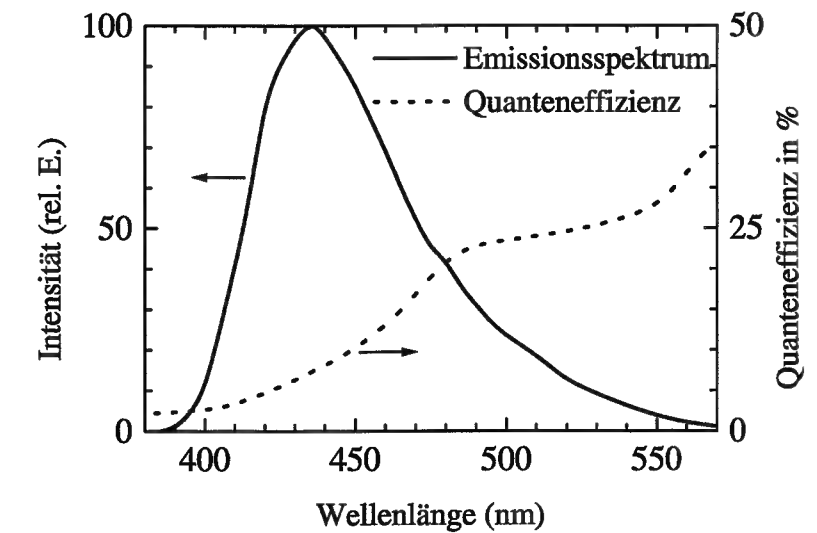
Abbildung 4.7: Emissionsspektrum der Fasern (durchgezogene Linie) und Quanteneffizienz des CCD-Chips (gestrichelte Linie). Die Pfeile deuten auf die Ordinate der jeweiligen Kurve.
