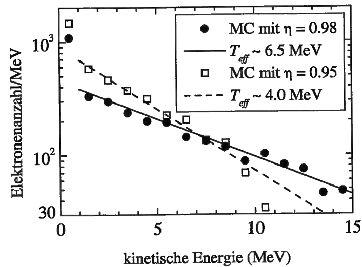
Abbildung 6.7: Energieverteilung der Elektronen und angepaßte Exponentialkurven der Monte-Carlo-Simulation mit T_{eff0} = 50 keV für \eta = 0.98 (gefüllte Punkte und durchgezogene Linie mit T_{eff} \sim 6.5 MeV) und 0.95 (offene Quadrate und gestrichelte Linie mit T_{eff} \sim 4.0 MeV) im Meßbereich des Spektrometers.
