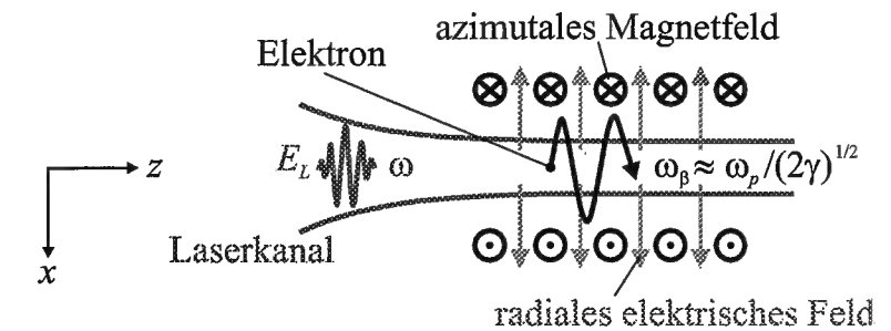
Abbildung 2.11: Schematische Darstellung der direkten Laserbeschleunigung. Das Elektron oszilliert mit der Betatronfrequenz \omega_\beta in den statischen Feldern des Kanals und wird bei Resonanz mit der Frequenz \omega des elektrischen Laserfeldes E_L beschleunigt.
