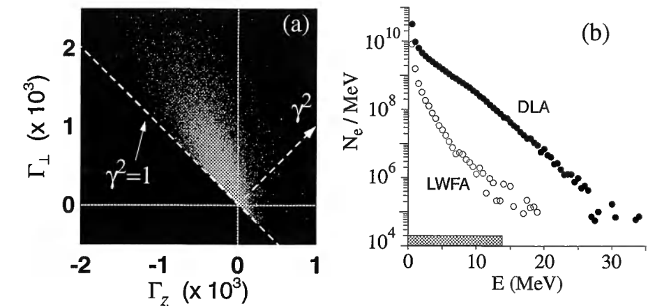
Abbildung 6.3: Aufschlüsselung des Elektronenspektrums der 3D-PIC-Simulation nach dem dominierenden Beschleunigungsmechanismus. (a) Verteilung der Elektronen in der (\Gamma_z, \Gamma_\perp) -Ebene. (b) Spektrale Verteilung der überwiegend durch DLA transversal beschleunigten Elektronen (gefüllte Punkte) bzw. der hauptsächlich durch LWFA longitudinal beschleunigten Elektronen (offene Punkte). Der Balken auf der Energieachse entspricht dem Meßbereich des Spektrometers.
