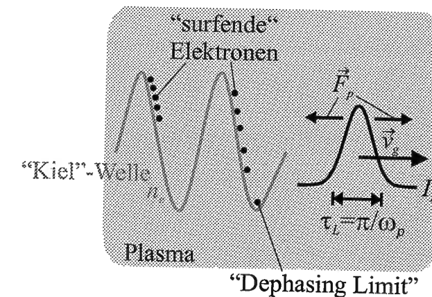
Abbildung 2.8: Schematische Darstellung der Wakefield-Beschleunigung: Die mit dem Intensitätsverlauf des Lasers I_L verbundene ponderomotorische Kraft \vec{F}_p regt eine Plasmawelle mit dem Dichteprofil n_e an, in der Elektronen beschleunigt werden, bis sie das Dephasing Limit erreichen.
