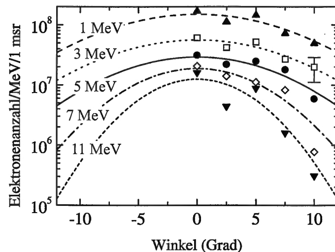
Abbildung 5.6: Winkeldivergenz von Elektronen der links angezeigten Energien ( n_e = 2 \times 10^{20} \text{ cm}^{-3} ). Symbole sind Meßdaten. Die Linien stellen angepaßte Gaußkurven (mit den Halbwertsbreiten - von oben nach unten - 16.5^\circ , 16^\circ , 14.6^\circ , 11.3^\circ und 9.3^\circ ) zur visuellen Hilfe dar, der Fehlerbalken resultiert aus Schuß-zu-Schuß Schwankungen.
