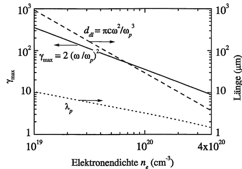
Abbildung 2.10: Maximal erreichbare Energie \gamma_{max} (durchgezogene Linie), Dephasing-Distanz d_{di} (gestrichelte Linie) und Plasmawellenlänge \lambda_p (gepunktete Linie) in Abhängigkeit von der Plasmadichte bei LWFA (für \lambda = 790 \text{ nm} ). Die Pfeile deuten auf die Ordinate der jeweiligen Kurve.
