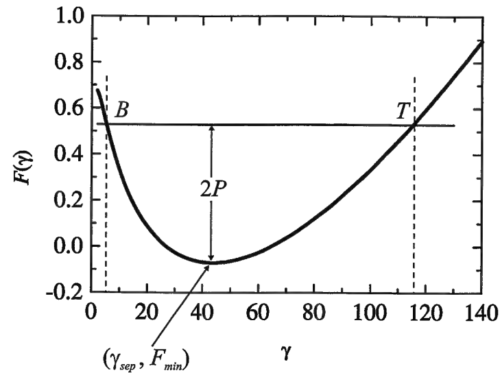
Abbildung 2.13: F als Funktion von \gamma (Gl. 2.62) für a_0 = 3 , n_0 = 2 \times 10^{20} \text{ cm}^{-3} und v_{xA} = 0.2 c . Die Energie zu dem Punkt B entspricht dem Minimum, die zu T dem Maximum der Separatrix in Abb. 2.14. Bei \gamma_{sep} treten die Schnittpunkte der Separatrix auf.
