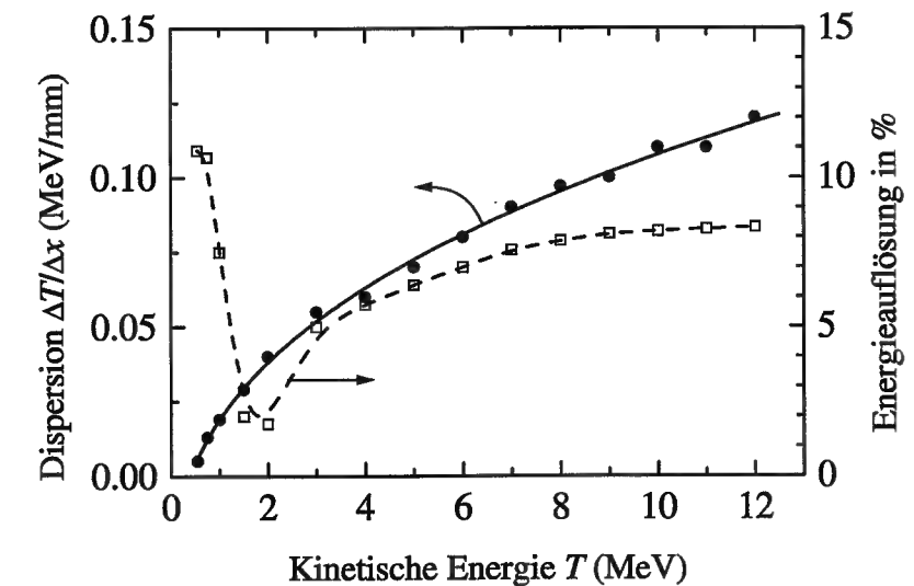
Abbildung 4.5: Dispersion (Ray-Tracing Ergebnisse dargestellt als Punkte, Fit als durchgezogene Linie) des Spektrometers und Energieauflösung bei Berücksichtigung der Blendenöffnung im Experiment (Quadrate und gestrichelte Linie). Die Pfeile deuten auf die Ordinate der jeweiligen Kurve.
