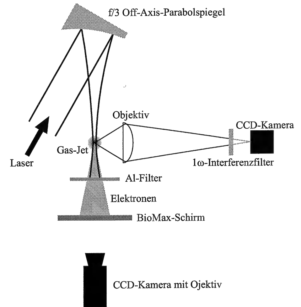
Abbildung 3.2: Experimenteller Aufbau zum Nachweis von Kanalbildung und MeV-Elektronen
