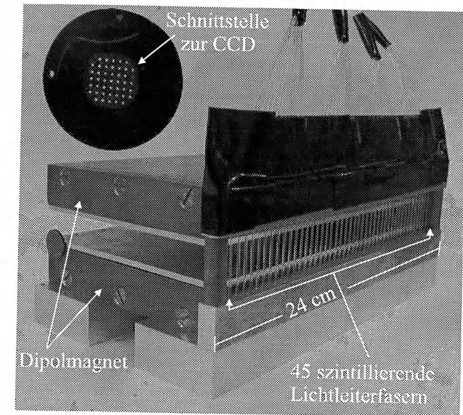
Abbildung 4.2: Photo des Elektronenspektrometers.
