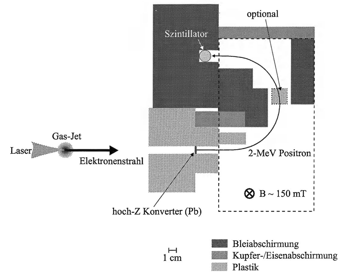
Abbildung 7.4: Experimenteller Aufbau zur Positronenerzeugung.
