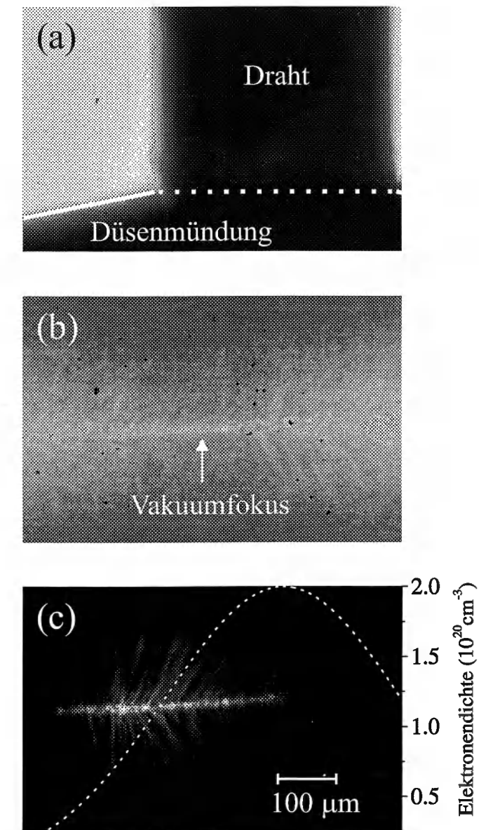
Abbildung 3.5: (a) Bestimmung der Position der Gasdüse, (b) Position des Vakuumfokus (c) Kanalbildung (Dichteprofil als gestrichelte Linie).
