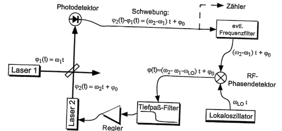
Fig. 4.8: Prinzip des optischen Phasenregelkreises. Im stabilisierten Zustand wird die integrale Größe Phase \varphi(t) = (\omega_2 - \omega_1 - \omega_{LO})t + \varphi_0 konstant gehalten. Für die Frequenz gilt damit \omega_2 = \omega_1 + \omega_{LO} . Momentane Phasenabweichungen \Delta\varphi führen bei der differentiellen Größe \omega in der Meßzeit \tau nur zu einem Fehler \Delta\omega \approx \Delta\varphi/\tau .
