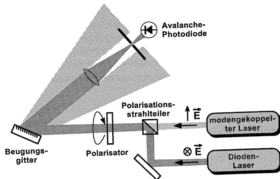
Fig. 4.9: Rauscharme Detektion eines Schwebungssignals mit dem modengekoppelten Laser auf einer Si Avalanche Photodiode. Die Strahlen der beiden Laser werden auf einem Polarisations-Strahlteiler mit orthogonaler Polarisation überlagert und anschließend mit einem drehbaren Polarisator auf eine gemeinsame Polarisationsachse projiziert. Um mögliche Änderungen der Strahlrichtung zu verhindern und die Polarisation optimaler Beugung des Gitters auszunutzen, kann der drehbare Polarisator durch ein \lambda/2 -Plättchen und einen festen Polarisator ersetzt werden. In den meisten Fällen ist die gezeigte Blende nicht kritisch und kann die Fläche der Photodiode selbst sein.
