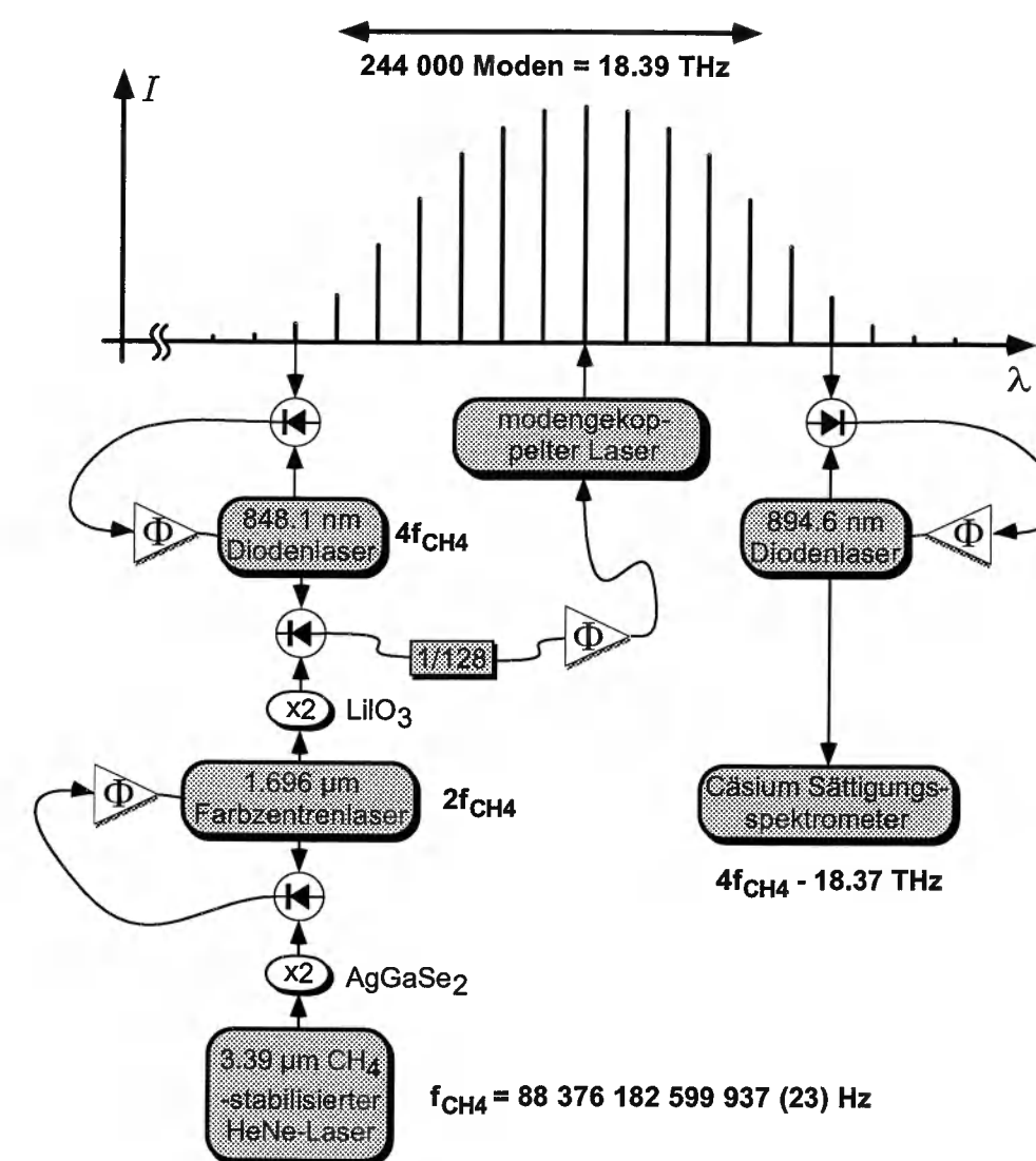
Fig. 5.2: Experimenteller Aufbau der Frequenzkette zur Messung der Cs- D_1 Linie. 244\,000 longitudinale Moden des modengekoppelten Lasers überbrücken das Frequenzintervall zwischen der D_1 Linie bei 894.6 \text{ nm} und 848.1 \text{ nm} , der vierten Harmonischen der genau bekannten Frequenz eines Methan-stabilisierten He-Ne-Lasers.
