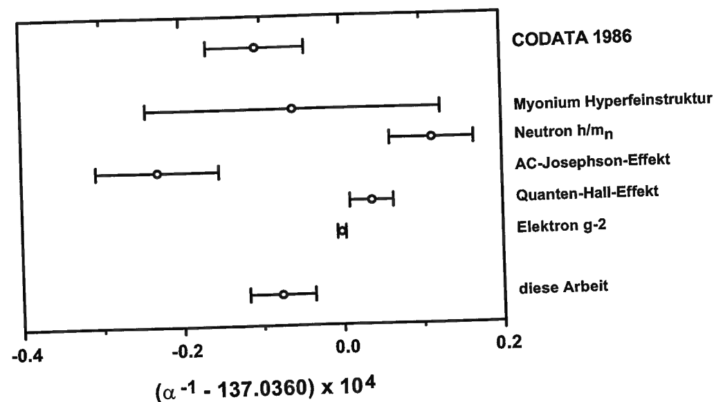
Fig. 5.1: Feinstrukturkonstante \alpha , aus verschiedenen Experimenten bestimmt. Zum Vergleich: Der in Codata 1986 [Cod87] veröffentlichte Wert. Die hier gezeigten Daten stammen aus [Kin96].
