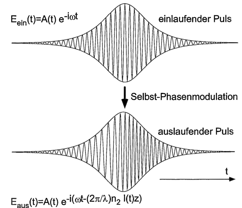
Fig. 3.3: Effekt der Selbst-Phasenmodulation auf einen Puls: Die Pulseinhüllende ändert sich (bei den hier erfolgten Näherungen) nicht. Die momentane Phase wird jedoch proportional zur momentanen Intensität verzögert. Erzeugung neuer Frequenzkomponenten an den Flanken ist die Folge.
