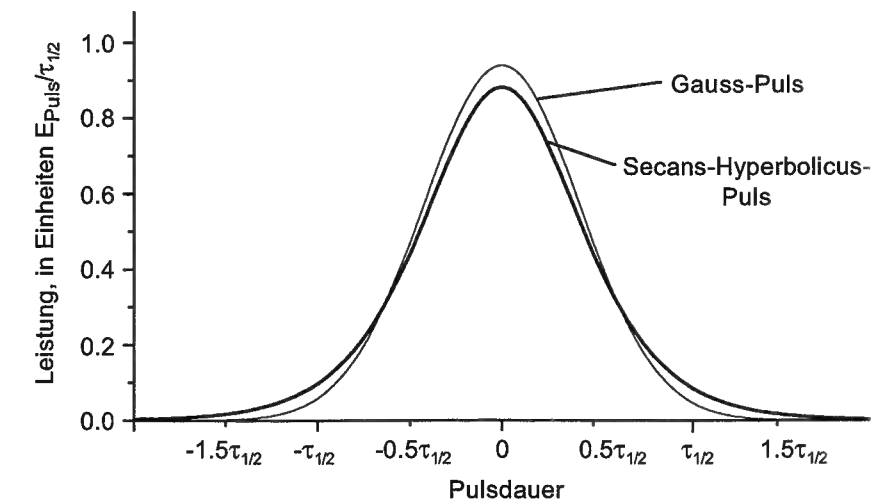
Fig. 3.4: Intensitätsprofil eines Secans-Hyperbolicus-Pulses im Vergleich zu einem Gauss-Puls gleicher Gesamtenergie E_{Puls} und gleicher Intensitäts-Halbwertsbreite \tau_{1/2} .
