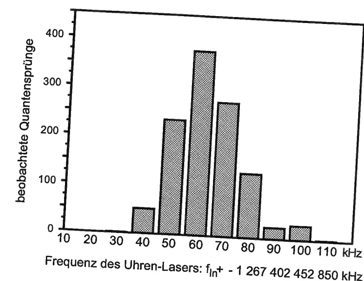
Fig. 7.4: Beobachtete Quantensprünge als Funktion der Absolutfrequenz des Uhren-Lasers (auf die Frequenz des \text{In}^+ -Übergangs hochgerechnet).
