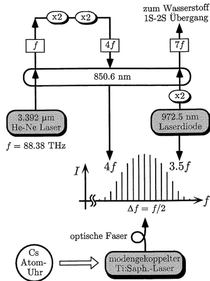
Fig. 1.1: Vereinfachtes Schema der neuen Frequenzkette zur Messung der 1S-2S Übergangsfrequenz in Wasserstoff bei 121.6 nm. Der optische Frequenzintervall-Teiler (ovales Symbol) legt das Verhältnis seiner Frequenzen auf f : 4f : 7f fest. Durch Messung der Frequenz eines stabilisierten He-Ne-Lasers in Form eines Intervalls der Größe f/2 bei 900 nm sind sämtliche Frequenzen im Versuchsaufbau bestimmt.
