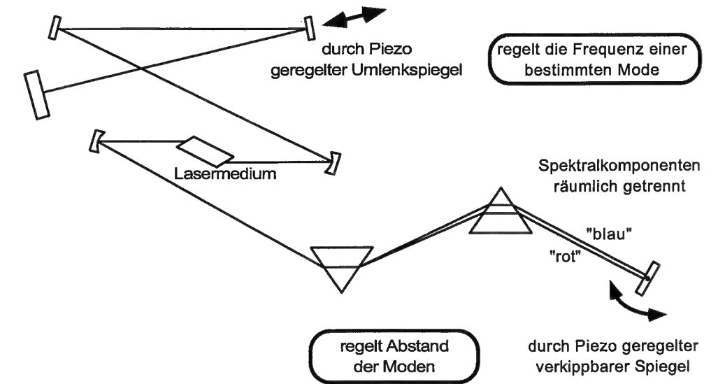
Fig. 4.3: Gleichzeitige Stabilisierung der beiden Parameter des Frequenzkamms, der Pulsrepetitionsrate und der Frequenz einer einzelnen Mode. Schnelle Regelung der Resonatorlänge stabilisiert die Frequenz einer bestimmten Mode. Langsameres Verkippen des Endspiegels ändert währenddessen die Pulsrepetitionsrate.
