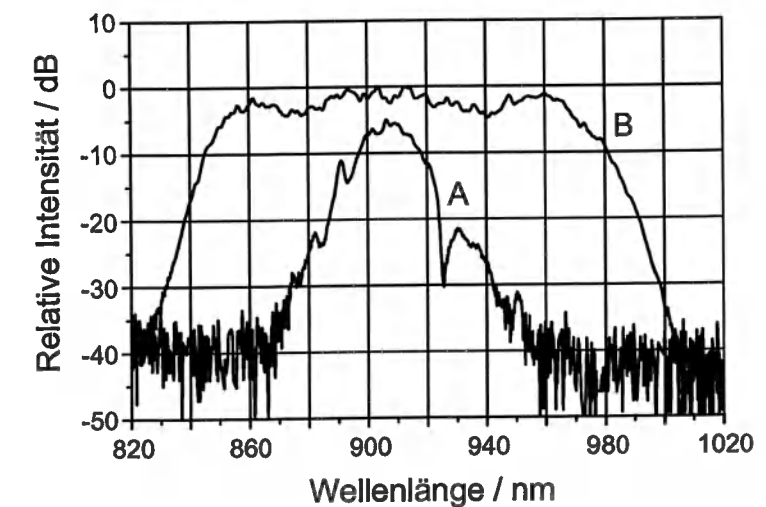
Fig. 4.5: Beobachtete spektrale Verbreiterung von 73 fs-Pulsen ( f_r = 76 MHz, 1.5-faches Pulsdauer-Bandbreite-Produkt) nach Passieren einer 40 cm langen optischen Ein-Moden-Faser. A: 8 mW des Ti:Saphir-Lasers eingekoppelt in die Faser; B: dieselbe Situation mit 225 mW mittlerer Leistung, gemessen am Faserausgang. Bei dem verbreiterten Spektrum können Laserdioden zuverlässig auf Moden phasenstabilisiert werden, deren Leistung weniger als -10 dB des Maximums beträgt.
