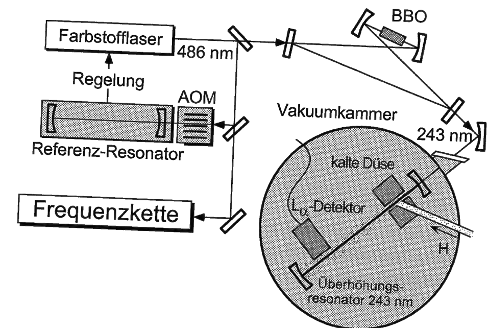
Fig. 6.5: Wasserstoff-Spektrometer zur Anregung der Doppler-freien 1S-2S Zweiphotonen-Resonanz bei \lambda = 243\text{ nm} . Metastabile 2S Atome werden mit einem elektrischen „Quenching“-Feld am L- \alpha -Detektor mit dem schnell zerfallenden 2P_{1/2} Zustand gemischt, wodurch sie ein Lyman- \alpha -Photon emittieren, das von einem Photomultiplier detektiert wird.
