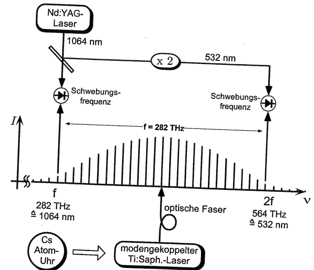
Fig. 8.1: Kompakte Frequenzkette auf Basis der Messung eines optischen Intervalls zwischen Laser-Harmonischen (Fundamentale f und zweite Harmonische 2f eines Nd:YAG-Lasers). Das Ausgangssignal eines Radiofrequenz-Synthesizers, der auf die Referenzfrequenz einer Cs-Atomuhr stabilisiert ist, wird mit Hilfe eines Femtosekundenlasers und nachfolgender spektraler Verbreiterung in einer optischen Faser in einem Schritt in eine optische Frequenz von 282 THz konvertiert (Radiofrequenz=Abstand der Moden des Frequenzkamms). Damit wird eine gesamte optische Oktave durch einen Kamm optischer Referenzfrequenzen überdeckt, die alle mit der relativen Genauigkeit der Radiofrequenz bekannt sind.
