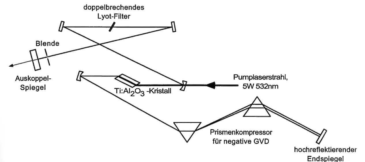
Fig. 4.2: Schematischer Aufbau eines mit Kerr-Linse modengekoppelten Festkörperlaserresonators, ähnlich dem in den Experimenten verwendeten Laser Modell Mira 900 (Coherent Inc.). Der Resonator ist ein linearer Resonator, cw-Moden erleiden durch eine Blende hohe Verluste. Die Gruppengeschwindigkeitsdispersion (GVD) des dispersiven Materials im Resonator wird mit einem prismatischen Kompressor kompensiert.
