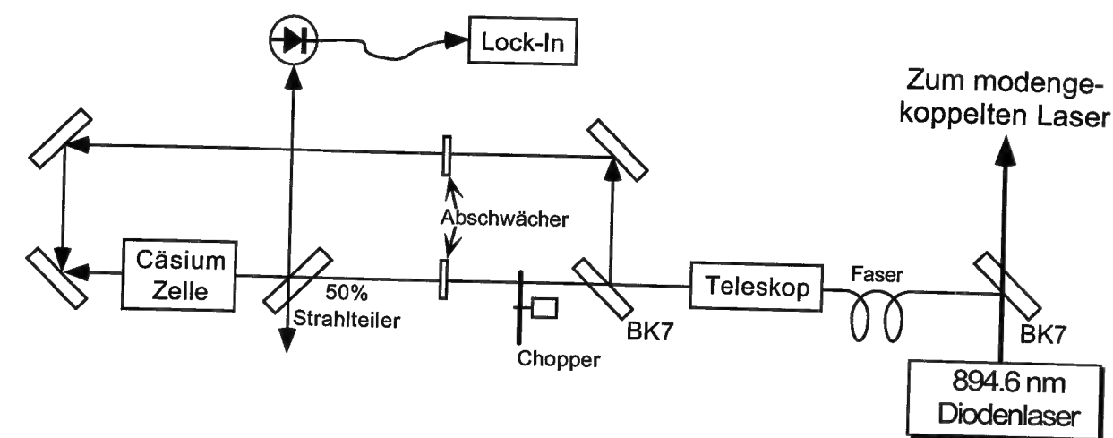
Fig. 5.3: Sättigungsspektrometer zur Doppler-freien Spektroskopie der D_1 Linie in Cäsium. Pump- und Probestrahl in kollinear Anordnung mit etwa gleichen Intensitäten.
