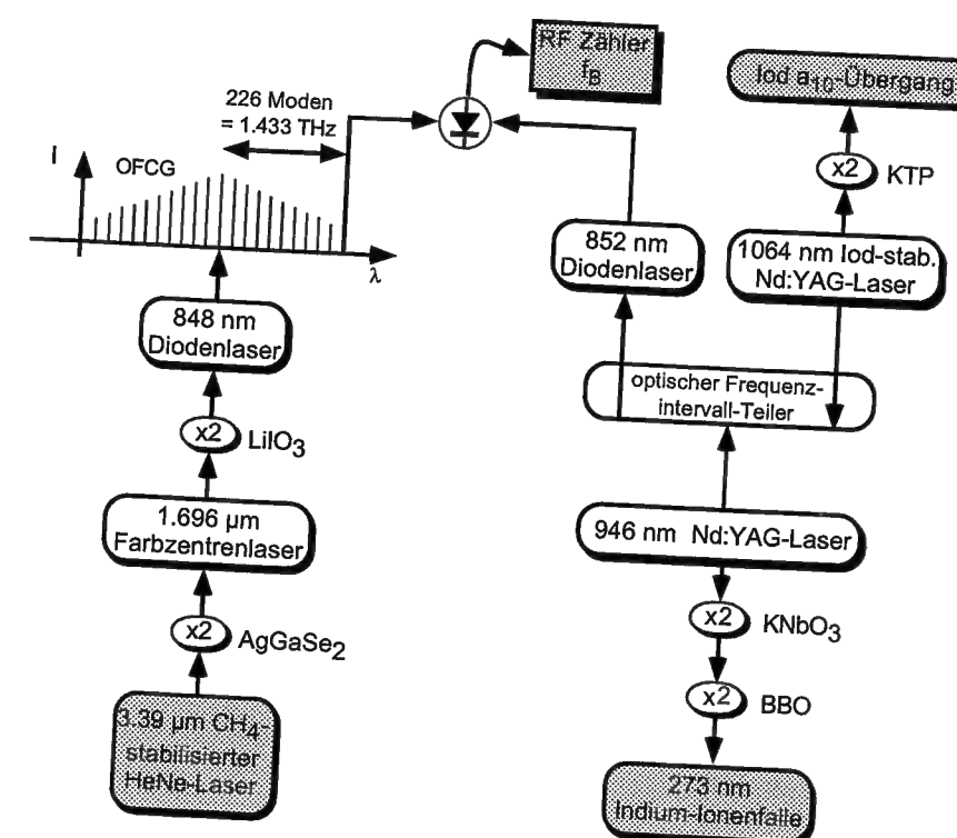
Fig. 7.3: Frequenzkette zur Messung der Frequenz 5s^2 1S_0 \rightarrow 5s5p^3 P_0 Übergangs. Die Frequenzkette verbindet die Frequenz von 88.4 THz eines Methan-stabilisierten He-Ne-Lasers bei 3.39 \mu\text{m} (links unten) und eines auf eine Iod-Linie bei 563 THz stabilisierten Nd:YAG-Lasers (1064 nm, rechts oben) phasenkohärent mit der Frequenz von 1 267 THz des Indium-Uhrenübergangs bei \lambda = 237 \text{ nm} (rechts unten). Eine Frequenzlücke von 1.433 THz wird von einem optischen Frequenzkamm-Generator (OFCG) überbrückt. Zur Bestimmung der Absolutfrequenz wird eine Schwebung f_B bei 852 nm mit einem Radiofrequenzzähler gezählt.
