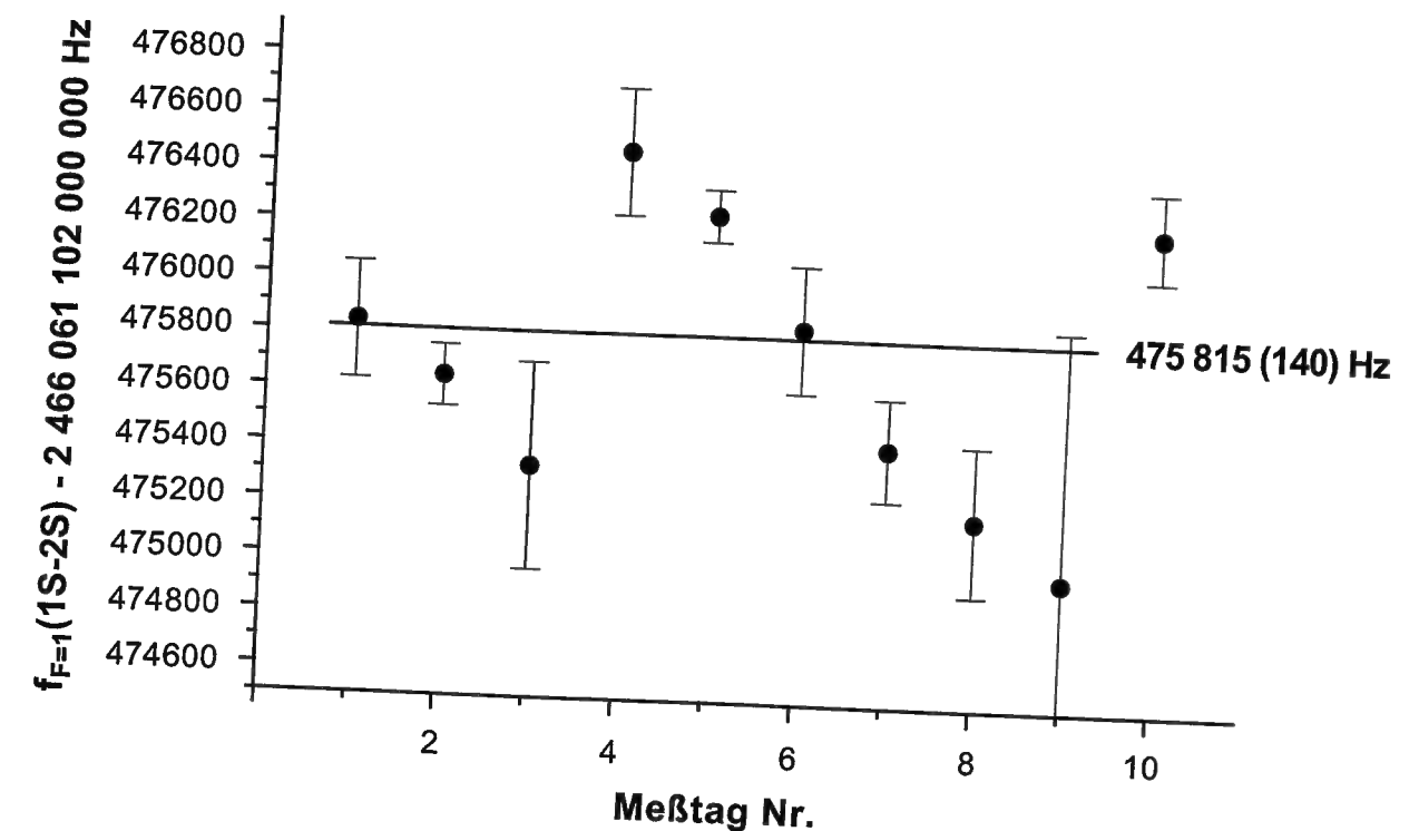
Fig. 6.9: Gesamtdaten der Messung des 1S_{1/2} (F=1) \rightarrow 2S_{1/2} (F'=1) -Intervalls in Wasserstoff. Gezeigt sind die Mittelwerte und Unsicherheiten der 10 Meßtage, in denen Unsicherheiten der Frequenz der Cs-Uhr noch nicht enthalten sind. Diese können aus der Streuung der Werte abgeschätzt werden. Systematiken des Wasserstoff-Spektrometers sind noch nicht korrigiert.
