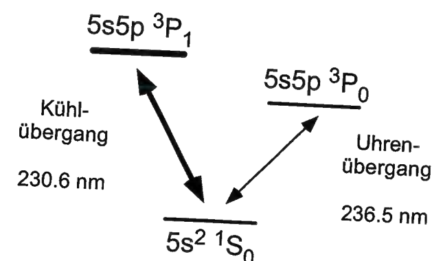
Fig. 7.1: Niedrigste Energieniveaus des \text{In}^+ -Ions. Das Ion wird durch Seitenbandkühlung auf der 5s^2 1S_0 \rightarrow 5s5p^3 P_1 Interkombinationslinie lasergekühlt (360 kHz natürliche Linienbreite). Anregungen auf dem „Uhrenübergang“ 5s^2 1S_0 \rightarrow 5s5p^3 P_0 mit weniger als 1 Hz Linienbreite werden durch fehlende Fluoreszenz des Kühlübergangs detektiert.
