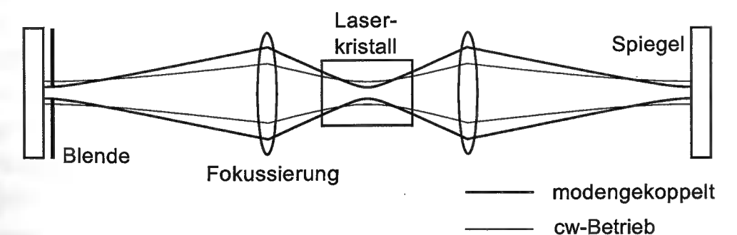
Fig. 4.1: Vereinfachte Darstellung eines Laserresonators zur Modenkopplung mit Kerr-Linse: Im modengekoppelten Betrieb auftretende Spitzenintensitäten bewirken durch Selbst-Fokussierung des Strahls im laseraktiven Material einen veränderten Strahlengang gegenüber dem cw-Betrieb. Eine Blende an geeigneter Stelle fügt höhere Verluste für cw-Moden ein und bevorzugt so den modengekoppelten Betrieb.
