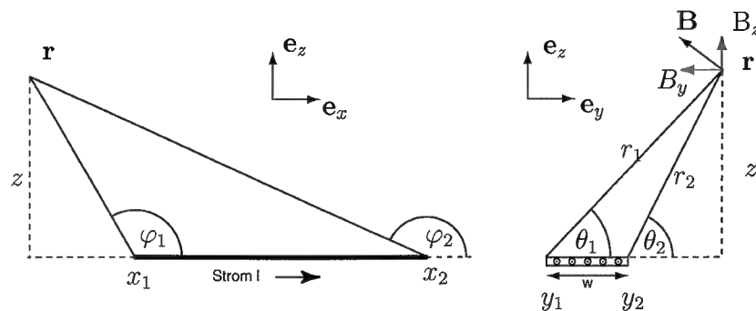
Abb. C.2: Breiter Draht
