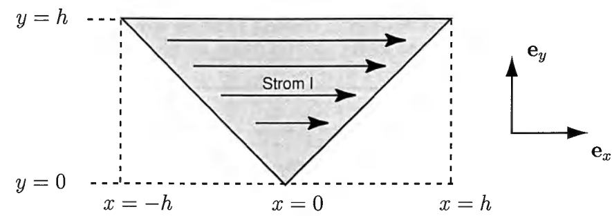
Abb. C.3: Dreiecksförmiges Verbindungsstück
