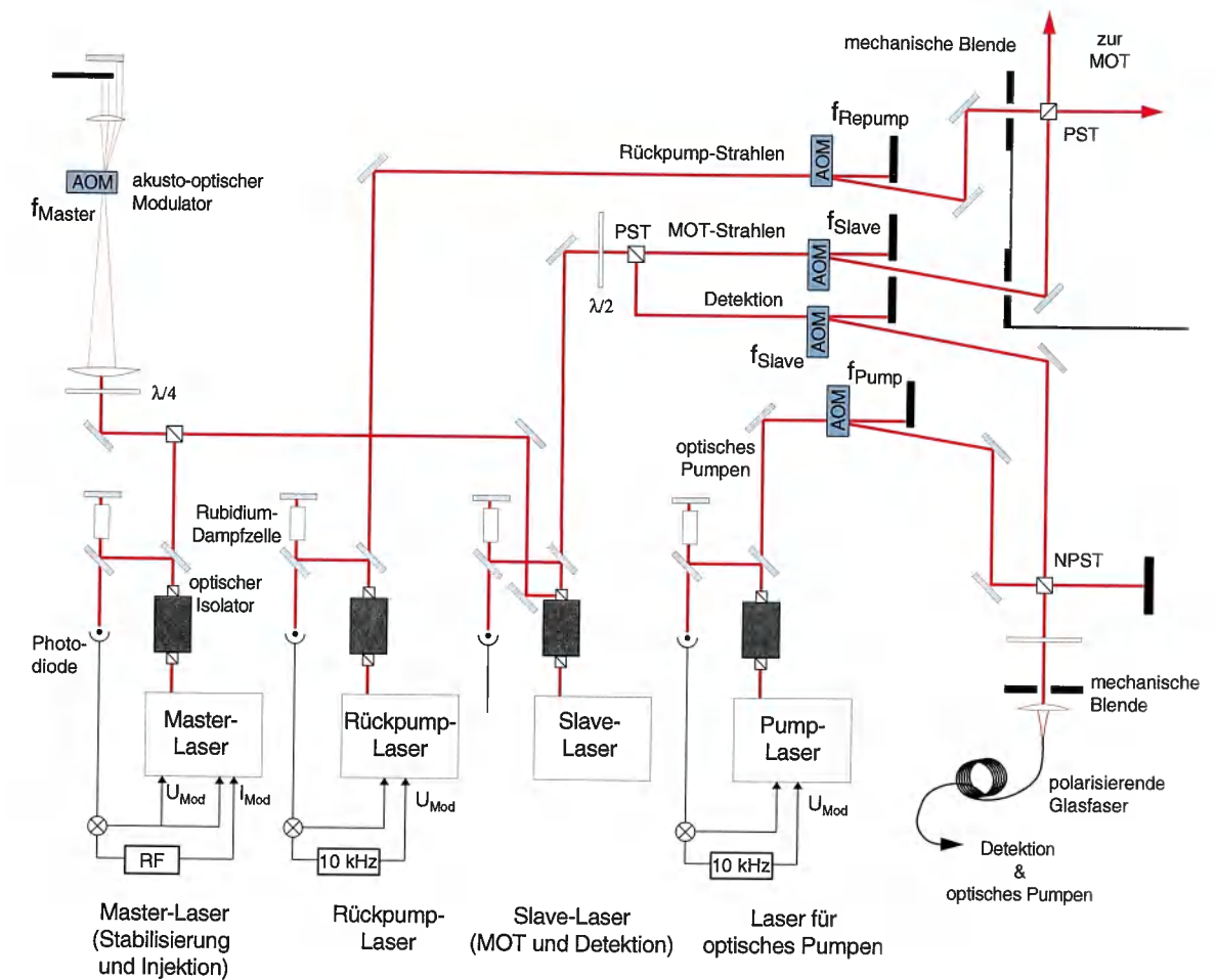
Abb. 4.10: Lasersystem:
