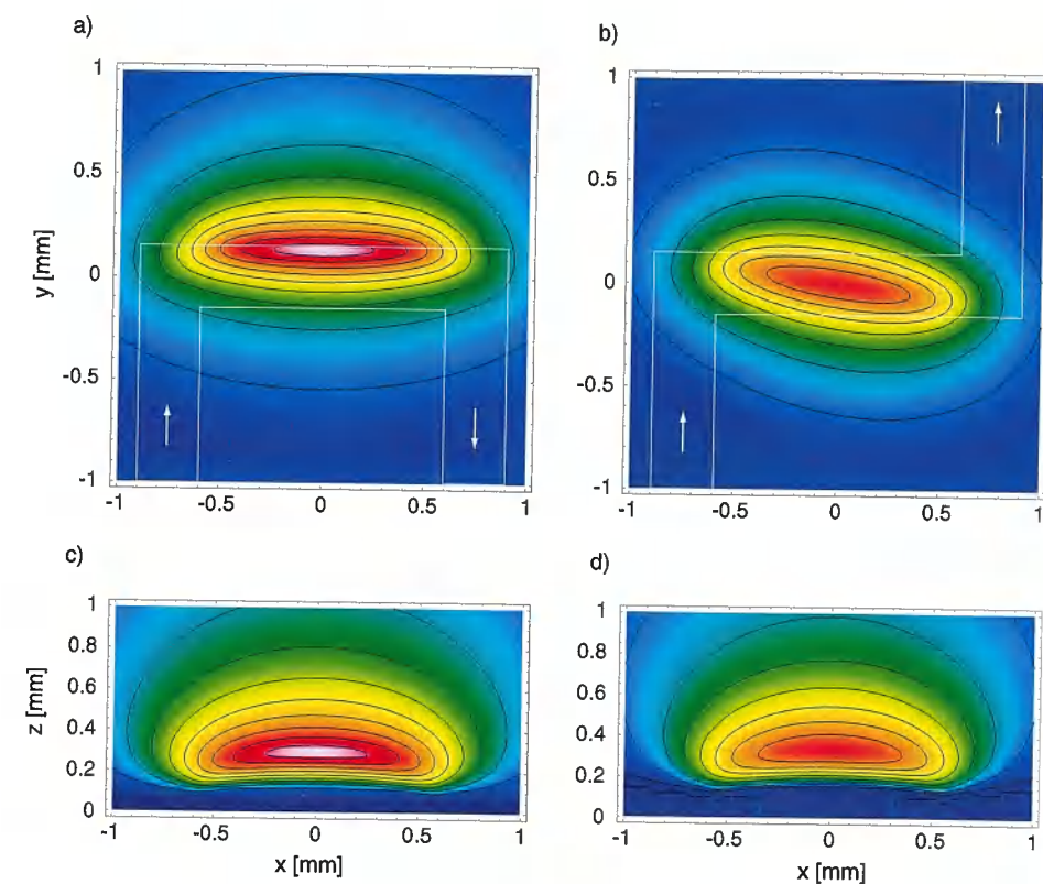
Abb. 3.18: Lage der Quadrupol- und Ioffe-Pritchard-Fallen am „u-förmigen“ und „z-förmigen“ Draht für I = 2\text{ A} , B_{0,y} = 10\text{ G} , Leiterbreite w = 300\text{ }\mu\text{m} und Abstand der Zuleitungen l = 1,5\text{ mm} . Die Höhenlinien markieren Feldstärken im Abstand von 1\text{ G} . Aufgetragen ist in jedem Punkt die minimale Feldstärke entlang der nicht sichtbaren Dimension (s. a. Anhang B.2).
