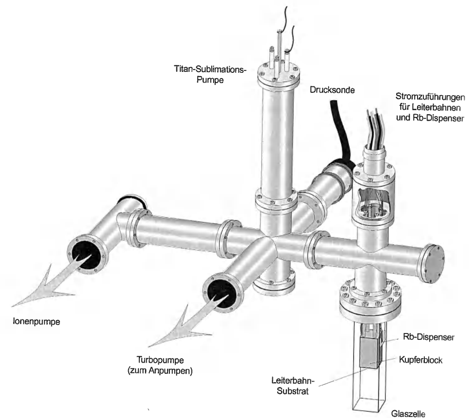
Abb. 4.9: Aufbau der Vakuumapparatur:
