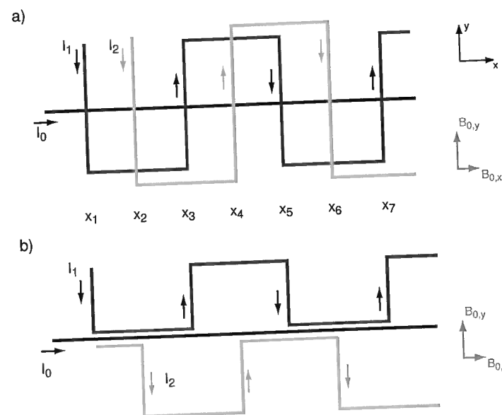
Abb. 3.20: Beim magnetischen Förderband entstehen die Fallenminima – anders als bei der „u-förmigen“ oder „z-förmigen“ Falle – über den stromführenden kreuzenden Drähten. Sehr günstig ließe sich ein Förderband realisieren, wenn sich verschiedene Leiterbahnen überkreuzen können (a). Für den Einsatz eines einlagigen Leiterbahnsubstrats müssen die quer verlaufenden Drähte die Kreuzung meiden (b), so daß die Schleifen aus a) jeweils auf eine Seite beschränkt sind.
