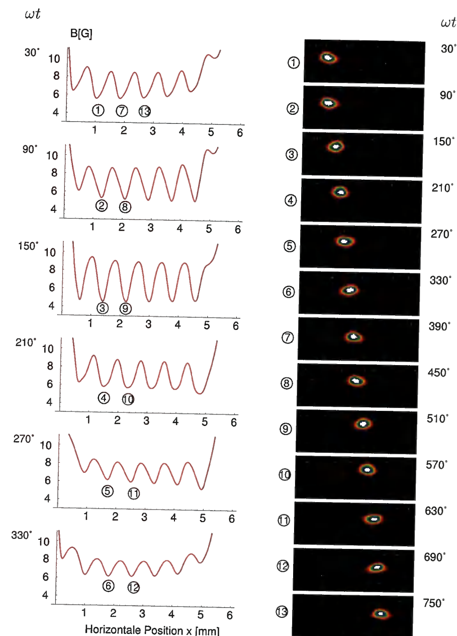
Abb. 5.15: Eine Kette von Ioffe-Pritchard-Fallen transportiert in einem ihrer Minima eine Atomwolke 4 \text{ mm} weit. Die Absorptionssbilder in der rechten Spalte zeigen zwei der insgesamt fünf Schiebezyklen. Links sind die zugehörigen Feldstärken aufgetragen, wie sie sich jeweils im Minimum senkrecht zur Transportrichtung ergeben.
