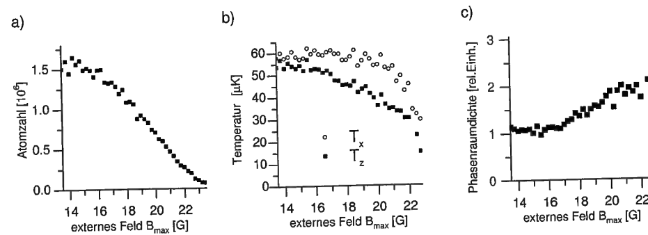
Abb. 5.11: Evaporatives Kühlen an der Oberfläche: Je näher die Atomwolke an das Substrat herangeführt wird, desto mehr heiße Atome werden durch den Kontakt mit der Oberfläche aus der Falle getrieben (a). Durch anschließende Thermalisation nimmt die Temperatur ab (b) und die Phasenraumdichte wächst (c).
