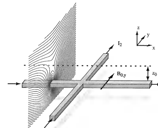
Abb. 3.7: Geometrie des Drahtkreuzes. Ist der Strom I_1 größer als I_2 , so läßt sich die entstehende Magnetfalle als Überlagerung des 2D-Quadrupols über Draht 1 mit dem Feld des senkrechten Drahtes interpretieren.
