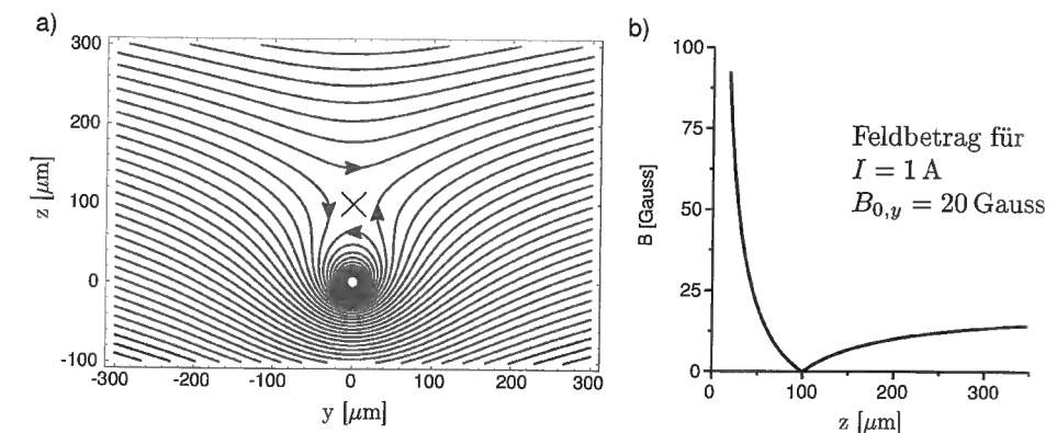
Abb. 3.4: Aus dem Magnetfeld des Drahtes ( I = 1 \text{ A} ) entsteht bei der Überlagerung mit dem konstanten Feld B_{0,y} = 20 \text{ G} ein zweidimensionales Quadrupolfeld mit Zentrum über dem Draht (a). Entlang der z -Achse besitzt der Feldbetrag eine Nullstelle mit unstetiger Ableitung (b).
