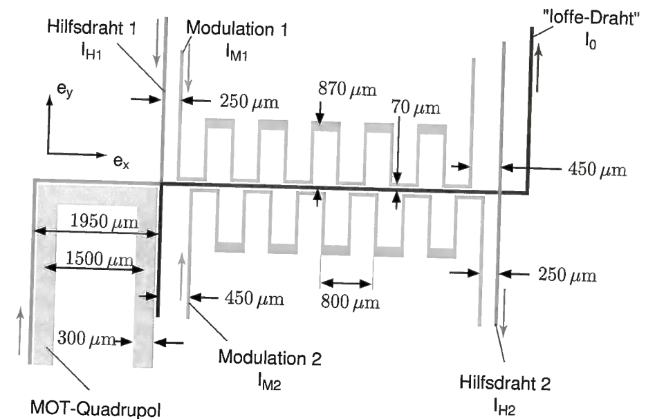
Abb. 5.12: Mikrofallensubstrat für das magnetische Förderband. Mit Ausnahme des u-förmigen Drahtes für die letzte Spiegel-MOT-Phase besitzen alle Leiterbahnen eine Breite von 50 \mu\text{m} , die markierten Abstände zwischen verschiedenen Leiterbahnen verstehen sich von Zentrum zu Zentrum. Die Flußrichtung, auf die sich Stromangaben im Text beziehen, ist durch schattierte Pfeile gekennzeichnet.
