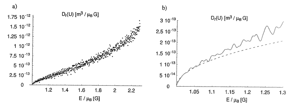
Abb. 3.15: Zustandsdichte D_f(U) im linken Potentialtopf, die durchgezogene Linie in b) zeigt die numerisch berechneten Werte aus a) nach einer Glättung. Nahe am Minimum folgt die Zustandsdichte dem wurzelförmigen Verlauf, den man für ein dreidimensionales harmonisches Potential erwartet (gestrichelte Linie).
