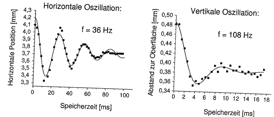
Abb. 5.8: Oszillationen in der Quadrupolfalle bei einem Strom von I = 2\text{ A} und einem externen Feld von B_{0,y} = 7,8\text{ G} . Aufgetragen ist jeweils der Schwerpunkt der Atomwolke gegen die Zeit.
