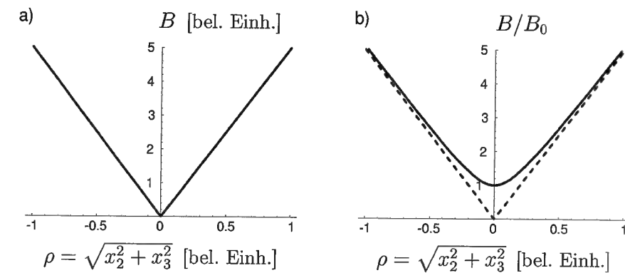
Abb. 2.4: Das transversale Profil der 2D-Quadrupolfalle (a) kann durch die Überlagerung mit einem konstanten Feld B_0 e_1 entlang der Symmetrieachse zu einem Feld transformiert werden, welches im Minimum nicht zu null wird (b).
