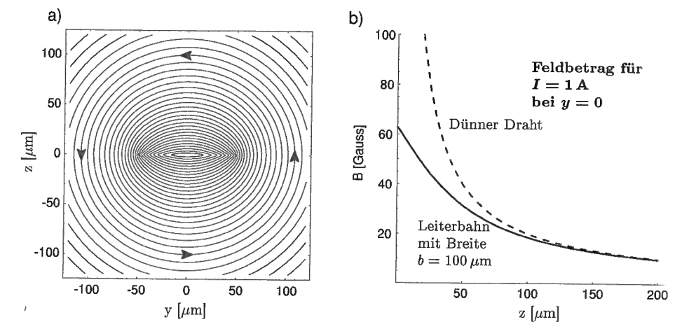
Abb. 3.5: a) Magnetfeldlinien einer 100\mu\text{m} breiten Leiterbahn, deren Höhe als unendlich gering angenommen ist, b) Feldstärke über dem Leiter bei einem Strom von 1 A: Die Abweichung vom Feld des unendlich dünnen Leiters wird deutlich, sobald der Abstand zum Leiter geringer wird als dessen Breite, der Feldbetrag an der Oberfläche beträgt etwa 62 G.
