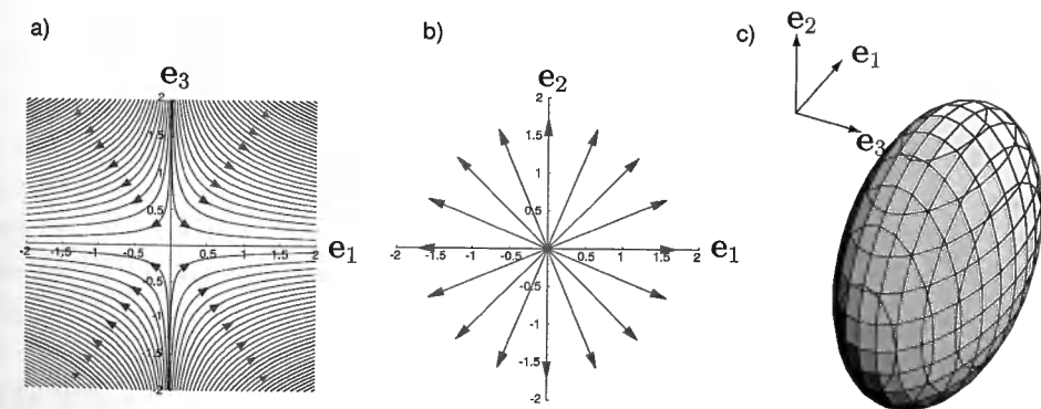
Abb. 2.2: a), b) Feldlinien des rotationssymmetrischen dreidimensionalen Quadrupols ( \alpha = \frac{1}{2} ). c) Die Flächen gleicher Magnetfeldstärke sind linsenförmige Ellipsoide um das Quadrupolzentrum (c).
