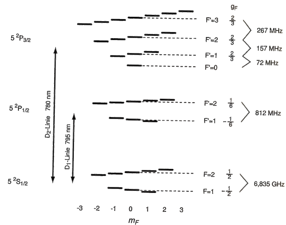
Abb. D.2: Termschema für ^{87}\text{Rb} (Kernspin I = 3/2 ). Die Aufspaltung der Unterzustände im Magnetfeld ist schematisch eingezeichnet.
