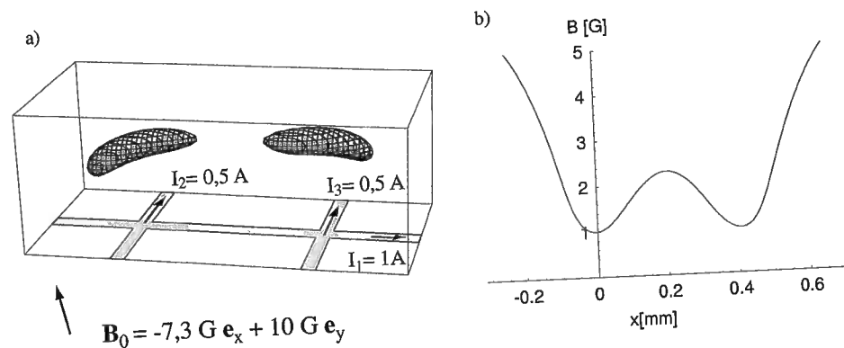
Abb. 3.14: Mit einem Hauptdraht und zwei kreuzenden Drähten läßt sich ein magnetisches Feld erzeugen, welches zwei Minima besitzt. a) Fläche konstanter Magnetfeldstärke B = 2 \text{ G} , b) Axialer Verlauf der Feldstärke nach der Minimum-Methode. Die beiden Fallen berühren sich bei einer Feldstärke von 2,3 \text{ G} .
