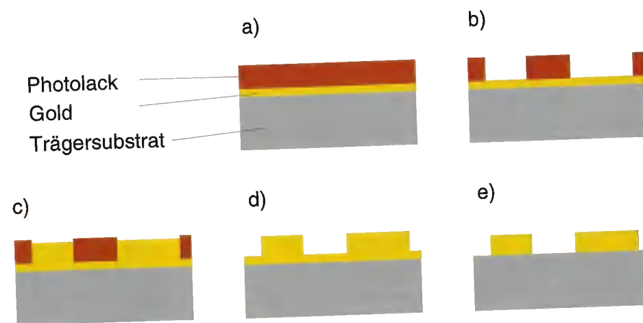
Abb. 4.3: Dünnschicht-Hybrid-Technik: Eine etwa 100 nm dünne Goldschicht wird an den durch Belichtung definierten Stellen galvanisch verstärkt (a-c). Anschließend wird auf der gesamten Fläche soviel Gold weggeätzt, daß die einzelnen Strukturen getrennt zurückbleiben (e).
