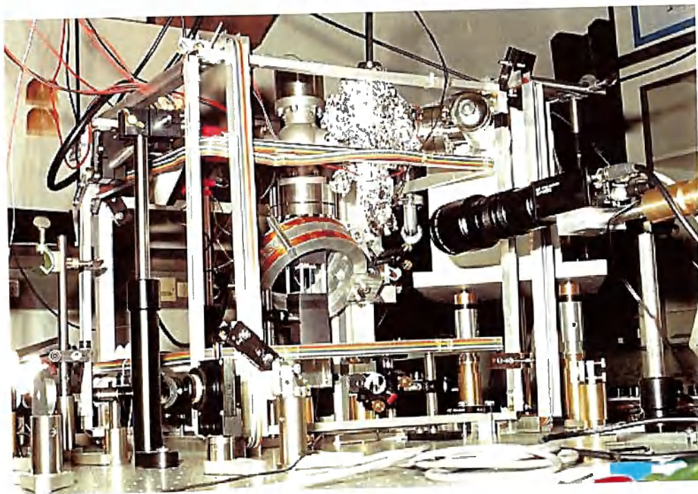
Abb. 4.2: Das Leiterbahnsubstrat hängt an einem Kupferträger von oben in eine Glaszelle. Das um 45^\circ geneigte Spulenpaar erzeugt das Quadrupolfeld für die magneto-optische Falle, die Atome werden mit der CCD-Kamera (rechts) über Absorptionsabbildung detektiert.
