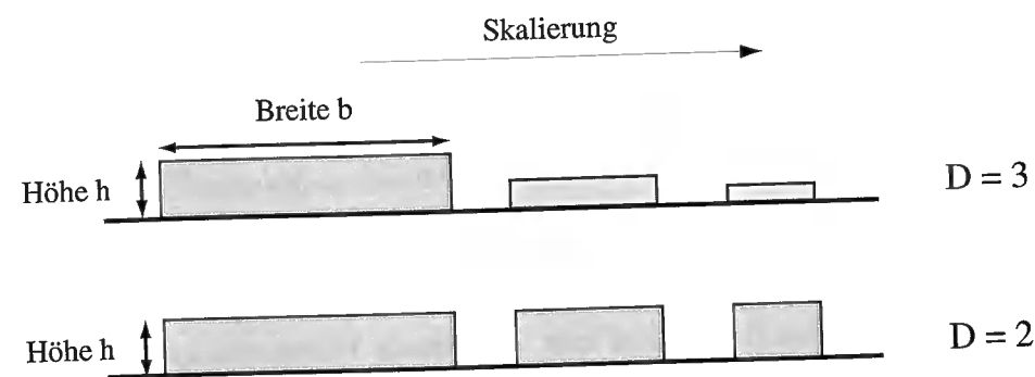
Abb. 3.24: Skalierung der Leitungsquerschnitte: Der dreidimensionalen Skalierung wird der Parameter D = 3 zugeordnet. Vor allem technische Bedeutung hat die zweidimensionale Skalierung D = 2 , bei welcher die Höhe der Struktur konstant gelassen wird.
