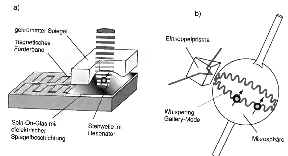
Abb. 6.2: a) Ein magnetisch gefangenes Atom koppelt in einem klassischen Resonator an das Lichtfeld, b) Zwei Atome werden in der Nähe einer Mikrosphäre durch das evaneszente Feld einer „Whispering-Gallery-Mode“ gekoppelt.
