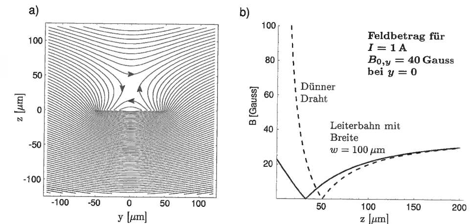
Abb. 3.6: a) Quadrupolfalle über einer 100\mu\text{m} breiten Leiterbahn. Entsteht die Falle in einer Entfernung von weniger als 100\mu\text{m} , so weicht der Verlauf der Feldlinien weniger vom Verlauf des idealen Quadrupols ab, als dies bei der Falle am unendlich dünnen Draht (Abb. 3.4) der Fall ist.
