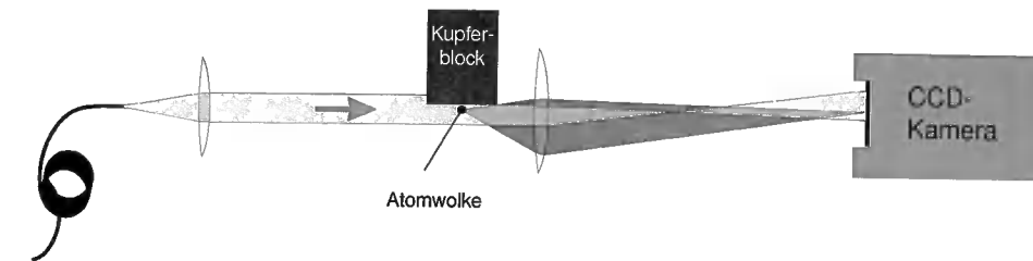
Abb. 4.11: Absorptionsabbildung in der Nähe der Substratoberfläche. Der Detektionsstrahl beleuchtet unter streifendem Einfall die Atome in der Mikrofalle. Der Schatten der Atome wird über ein Zoom-Objektiv (hier schematisch durch eine Linse angedeutet) auf eine CCD-Kamera abgebildet.
