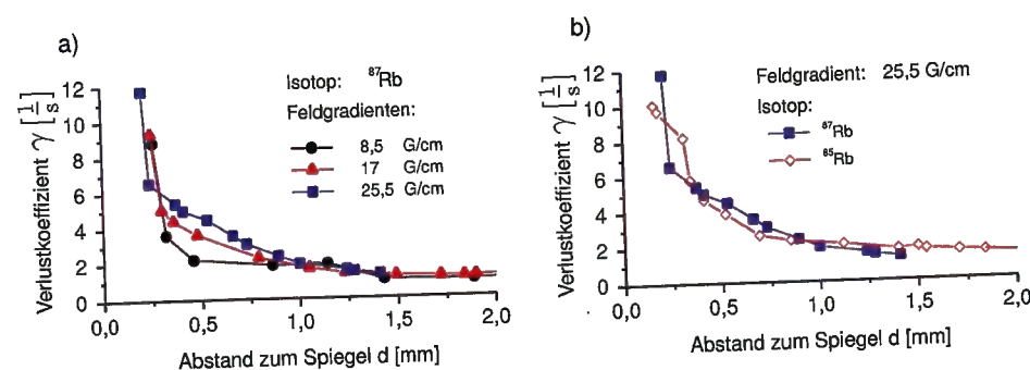
Abb. 5.1: Verlustrate in der Spiegel-MOT als Funktion des Abstands zum Spiegel: a) für verschiedene Gradienten, b) für die verschiedenen Isotope.
