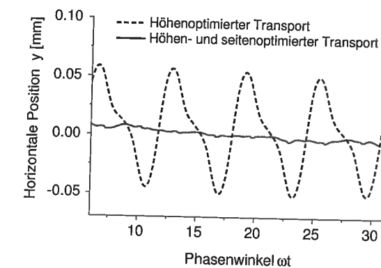
Abb. 5.18: Zeitlicher Verlauf des Schwerpunkts entlang der e_y -Achse. Die beim höhenoptimierten Förderband vorhandene Schwerpunktsbewegung (gestrichelt) läßt sich durch ein zusätzliches Magnetfeld entlang e_z reduzieren (b).
