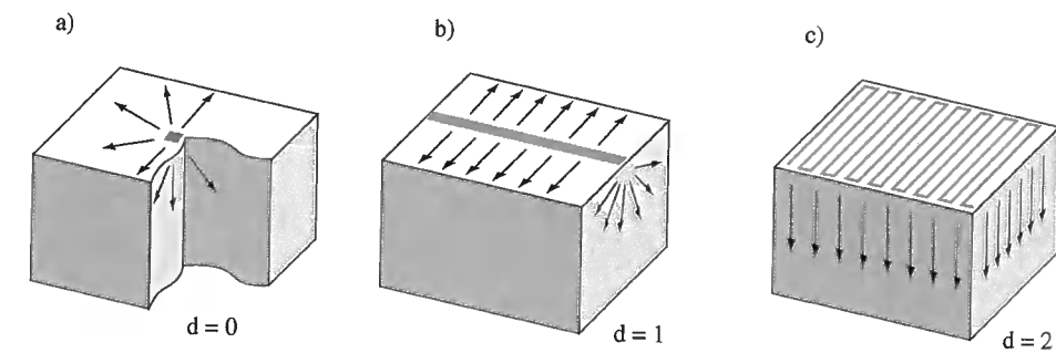
Abb. 3.22: Die Dimensionalität der Leiterstruktur ist ein zentraler Parameter bei der Skalierung von Mikrofallen. „0-dimensionale“ Strukturen verringern ihre wärmeerzeugende Fläche bei der Skalierung und ermöglichen eine dreidimensionale Wärmeableitung in das Substrat (a). Bei eindimensionalen Strukturen wie in b) ist die Wärmeleitung auf zwei Dimensionen reduziert, zweidimensionale Strukturen wie Atomspiegel oder parallel betriebene Magnetfallen (c) ermöglichen lediglich eindimensionalen Wärmetransport.
