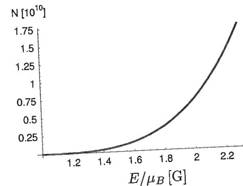
Abb. 3.16: Anzahl der Quantenzustände im linken Potentialtopf. Das lokale Minimum faßt 1,73 \cdot 10^{10} Quantenzustände für ^{87}\text{Rb} im |F=2, m_F=2\rangle -Grundzustand, bis die Falle bei B = 2,3 \text{ G} überläuft.
