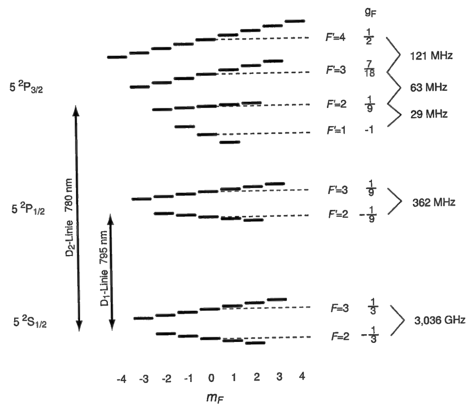
Abb. D.1: Termschema für ^{85}\text{Rb} (Kernspin I = 5/2 ). Die Aufspaltung der Unterzustände im Magnetfeld ist schematisch eingezeichnet.
