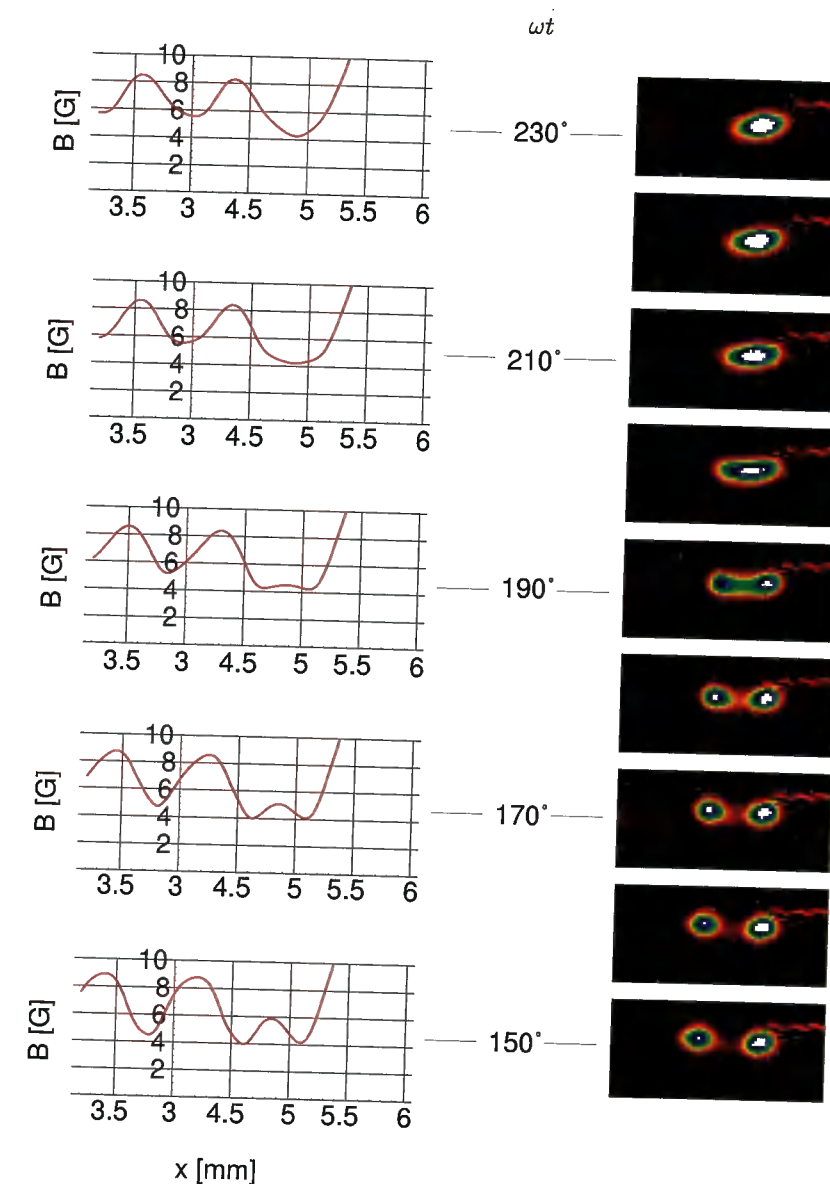
Abb. 5.24: Aufteilen der Ioffe-Pritchard-Falle
