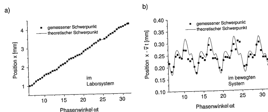
Abb. 5.19: Zeitlicher Verlauf des Schwerpunkts beim höhenoptimierten Förderband. a) x -Position im Laborsystem, b) x -Position im gleichförmig bewegten Bezugssystem.
