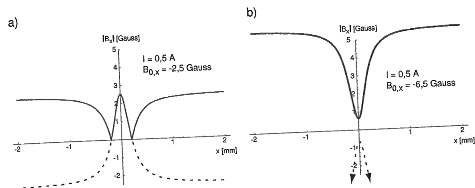
Abb. 3.10: Die Überlagerung des Drahtfeldes aus Abb. 3.8 mit einem homogenen Feld in e_x -Richtung führt dazu, daß entlang der e_x -Achse zwei Nullstellen auftreten (a) oder sich ein lokales Minimum bildet (b). An diesen Stellen führt die Überlagerung mit dem zweidimensionalen Quadrupol des ersten Drahtes zu zwei dreidimensionalen Quadrupolfallen bzw. zu einer Ioffe-Pritchard-Falle.
