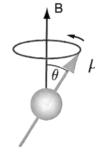
Abb. 2.1: Ist das magnetische Moment eines Teilchens an einen Drehimpuls gekoppelt, so präzidiert im Magnetfeld dieses Moment um die Feldachse.
