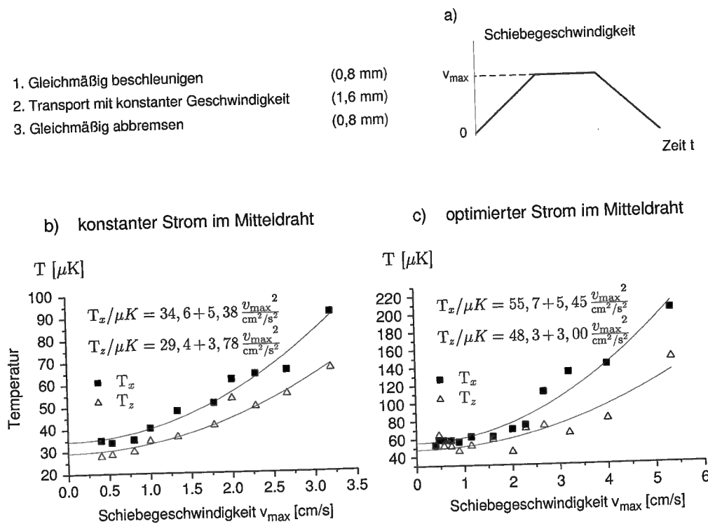
Abb. 5.17: a) Verlauf der Geschwindigkeit beim Transport über 4 Förderbandperioden, b) und c) Heizrate durch den Transport.
