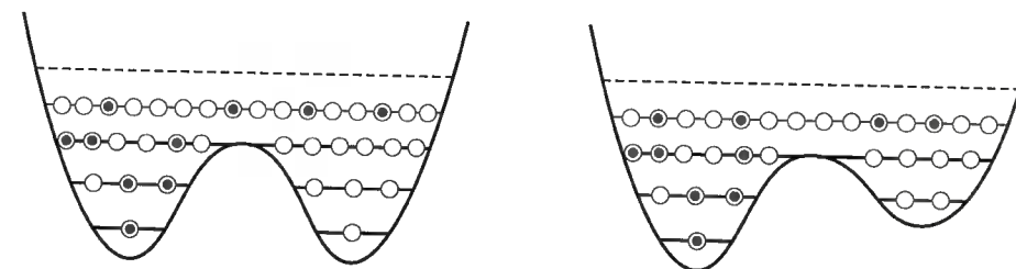
Abb. 5.20: Eine optimale Vereinigung findet statt, wenn die Besetzungswahrscheinlichkeit der Zustände an der Vereinigungskante in beiden Potentialen gleich groß ist.
