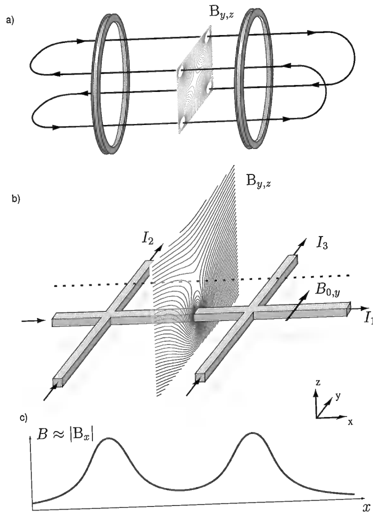
Abb. 3.9: a) Klassische Ioffe-Pritchard-Falle, b) Realisierung der Ioffe-Pritchard-Falle als Mikrofalle, c) Feldbetrag entlang der Quadrupolachse.
