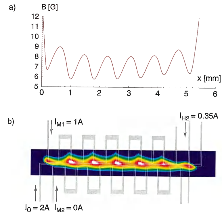
Abb. 3.21: Position der Minima beim atomaren Förderband. Die Felder sind berechnet für \mathbf{B} = 7 \text{ G} \mathbf{e}_x + 16 \text{ G} \mathbf{e}_y .
