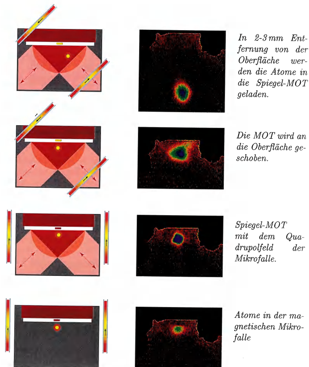
Abb. 5.3: Der Ladevorgang ist illustriert mit den ersten Bildern unserer magnetischen Mikrofalle. Die schematischen Ansichten (links) und die Absorptionsspektroskopie-Bilder (Mitte) zeigen die Position der Atomwolke aus zueinander senkrechten Richtungen. In den Skizzen verläuft der Sondenstrahl von links nach rechts.
