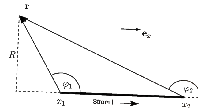
Abb. C.1: Dünner Draht
