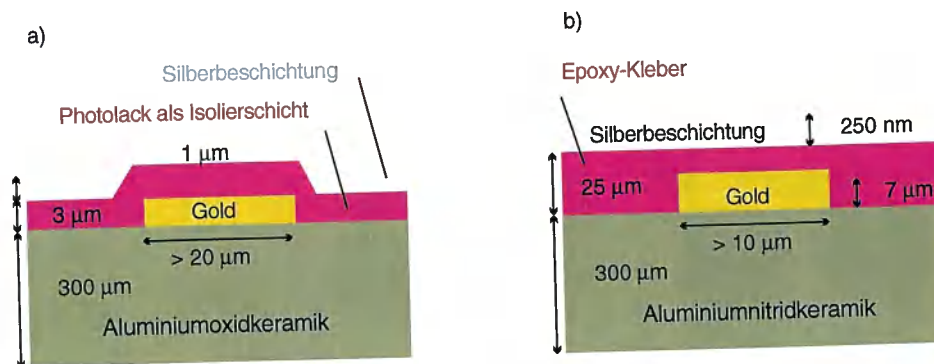
Abb. 4.5: a) Die ersten Mikrofallensubstrate spiegeln in ihrer Oberflächenstruktur die Struktur der Leiterbahnen wider. b) Die Substrate der „zweiten Generation“ werden mit der Technik der Replika-Optik verspiegelt, so daß die Oberfläche eben wird.
