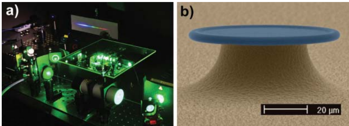
Abb. 3: Vergleich zwischen herkömmlichem Titan-Saphir Frequenzkammgenerator (a) und dem neuartigen Mikrotoroid-Frequenzkammgenerator aus Glas (b). In diesem Mikroskopbild ist die Glasstruktur mit blauer Farbe hervorgehoben. Laserlicht kann über eine Glasfaser in den Toroid eingekoppelt werden und wird dort durch fortlaufende Reflektion an der Innenwand gespeichert. Der Mikrotoroid ist etwa 10000-mal kleiner als ein Titan-Saphir Frequenzkammgenerator.
